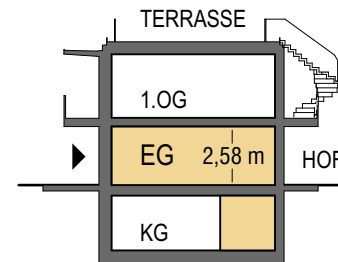
SCHNITT
